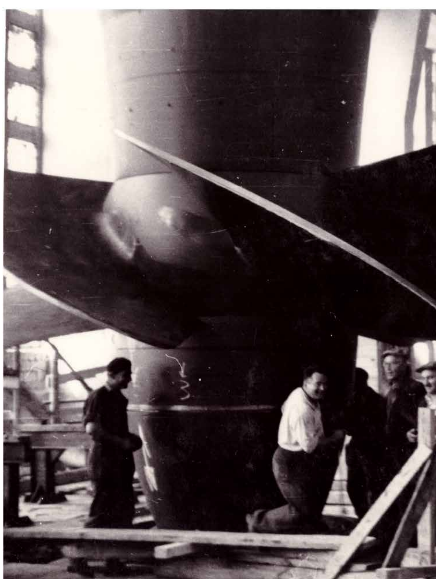
Priehradou spútaná sila Váhu roztáča lopatky Kaplanovej turbíny - srdce elektrárne, ktoré neúnavne generuje elektrickú energiu.
